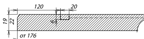
Сечение фасада
