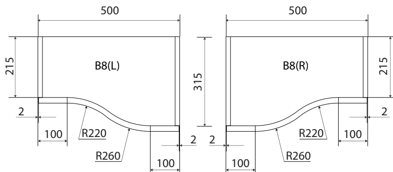
ВЕРХНИЙ МОДУЛЬ С S - ОБРАЗНЫМ ФАСАДОМ B8 МИН./МАКС ВЫСОТА, ММ: 496/1000
