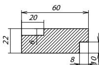
Сечение витрины
