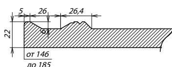
Сечение ПСЯ
