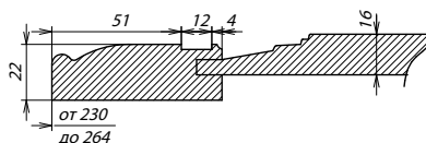
Сечение ПСЯ
