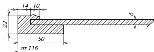
Сечение фасада
