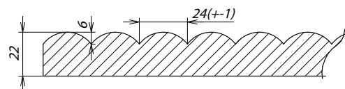
Сечение фасада
