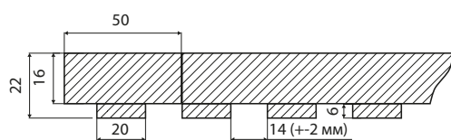
Сечение фасада
