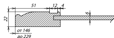
Сечение ПСЯ
