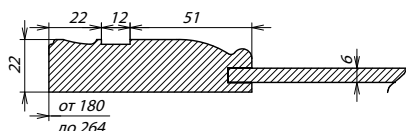
Сечение ПСЯ
