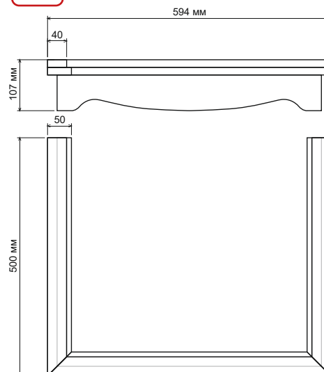
Схема вытяжки
