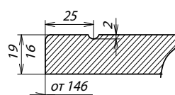
Сечение фасада S9, S10 (горизонтальная траверса)
