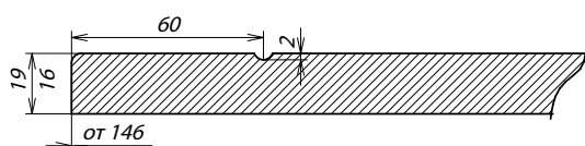
Сечение фасада S7, S8, S10 (вертикальная траверса)
