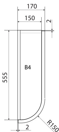
НИЖНИЙ МОДУЛЬ С ГНУТЫМ ФАСАДОМ B4 МИН./МАКС ВЫСОТА, ММ: 496/1500 (для S1)
