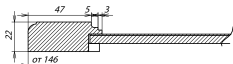
Сечение фасада
