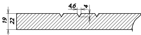
Сечение фасада
