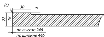
Сечение фасада
