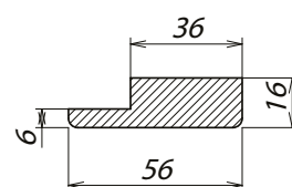
Планка торцевая Т2
