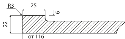
Сечение фасада
