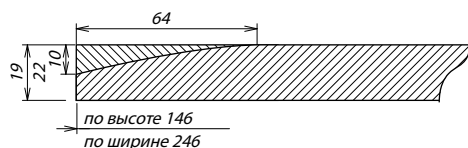
Сечение фасада
