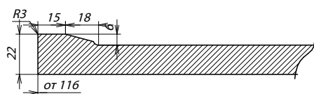
Сечение фасада
