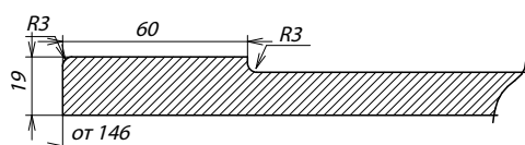
Сечение фасада
