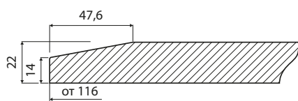
Сечение фасада
