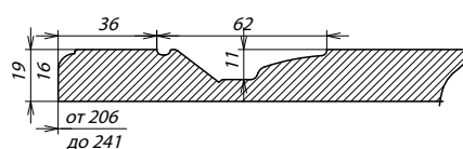
Сечение ПСЯ
