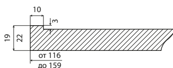
Сечение ПСЯ
