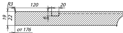
Сечение фасада
