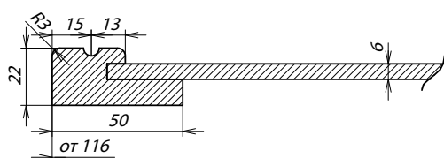
Сечение фасада
