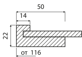
Сечение фасада
