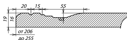
Сечение ПСЯ
