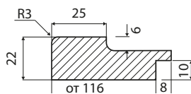
Сечение витрины
