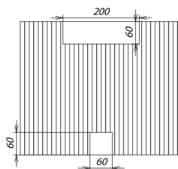
Схемы выборки под ручки
