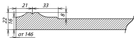
Сечение фасада
