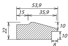
Сечение витрины
