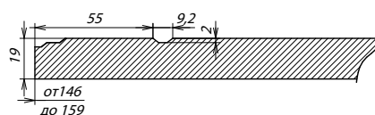
Сечение ПСЯ
