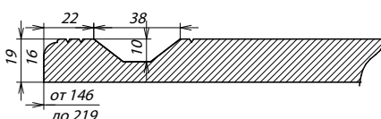
Сечение ПСЯ
