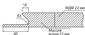
Сечение фасада
