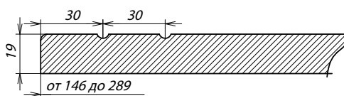
Сечение ПСЯ
