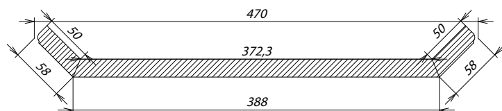
Схема трапеции
