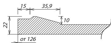
Сечение фасада
