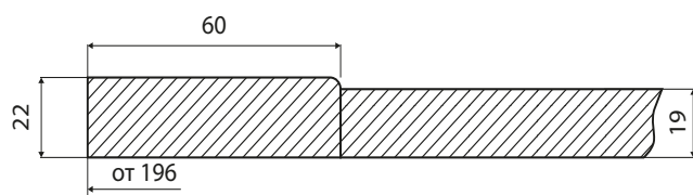
Сечение фасада
