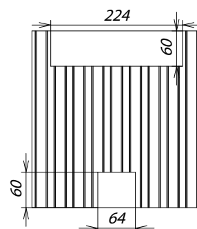
Схемы выборки под ручки
