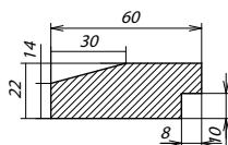
Сечение витрины
