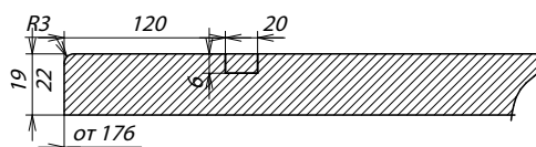
Сечение фасада
