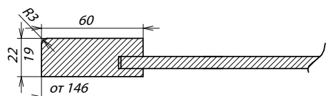
Сечение фасада
