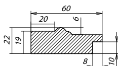
Сечение витрины
