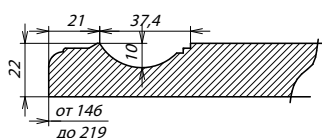
Сечение ПСЯ
