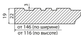
Сечение фасада
