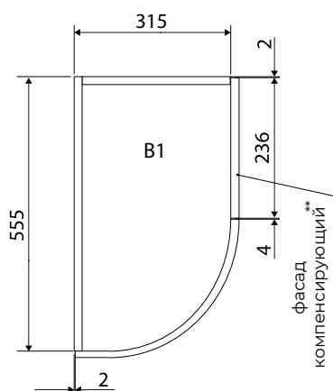
ВЕРХНИЙ МОДУЛЬ С ГНУТЫМ ФАСАДОМ В1 COLOR: МИН./МАКС ВЫСОТА, ММ: 360/2450 (ДЛЯ S1, W1, D1) DECOR: МИН./МАКС ВЫСОТА, ММ: 360/1600 (ДЛЯ S1)
