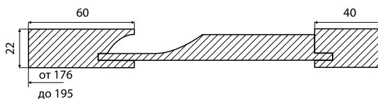
Сечение ПСЯ
