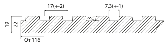
Сечение фасада
