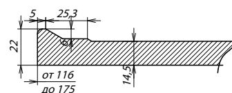
Сечение ПСЯ
