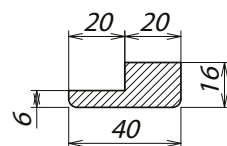
Планка торцевая Т1
