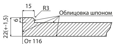
Сечение фасада
