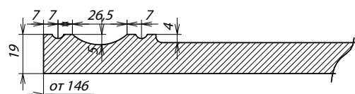
Сечение фасада
