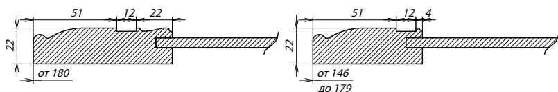
Сечение фасада
