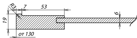
Сечение фасада
