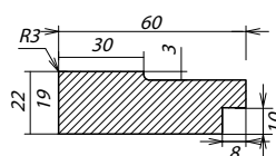
Сечение витрины
