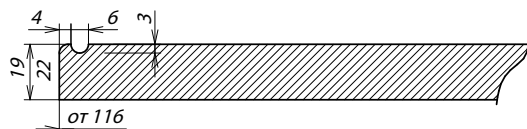
Сечение фасада
