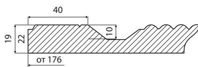
Сечение фасада
