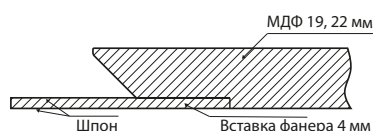
Сечение фасада
