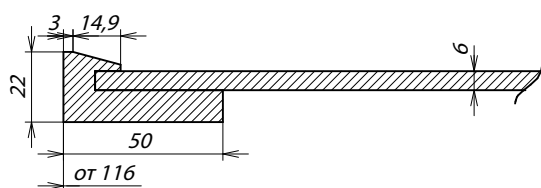
Сечение фасада
