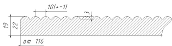
Сечение фасада
