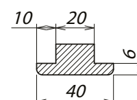
Планка стыковочная
