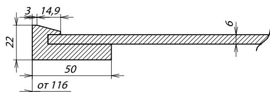
Сечение фасада
