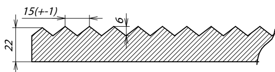
Сечение фасада
