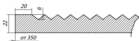
Сечение фасада
