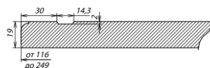
Сечение ПСЯ
