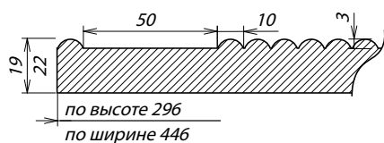
Сечение фасада
