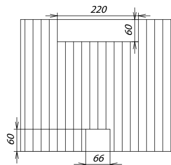
Схемы выборки под ручки
