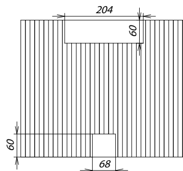
Схемы выборки под ручки
