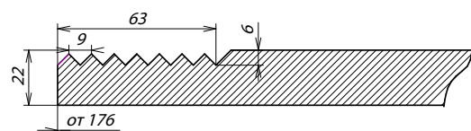
Сечение фасада
