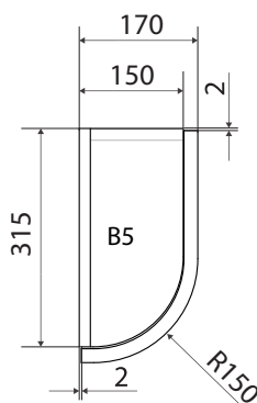
ВЕРХНИЙ МОДУЛЬ С ГНУТЫМ ФАСАДОМ B5 МИН./МАКС ВЫСОТА, ММ: 496/1500 (для S1)
