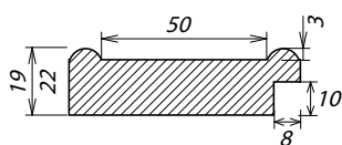
Сечение витрины
