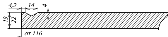
Сечение фасада
