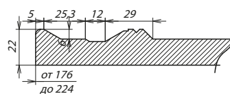
Сечение ПСЯ
