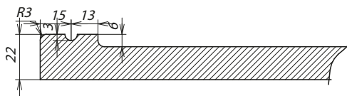
Сечение фасада
