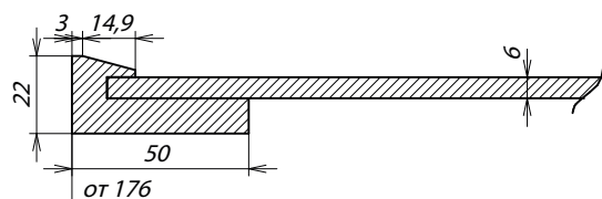
Сечение фасада
