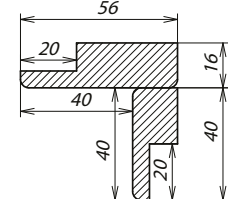
Угловое соединение торцевых планок
