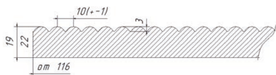
Сечение фасада
