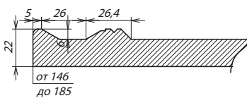
Сечение ПСЯ
