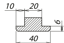
Планка стыковочная
