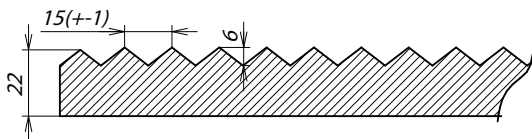
Сечение фасада
