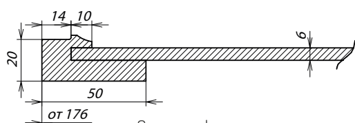
Сечение фасада
