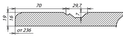
Сечение фасада
