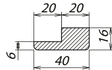
Планка торцевая T1
