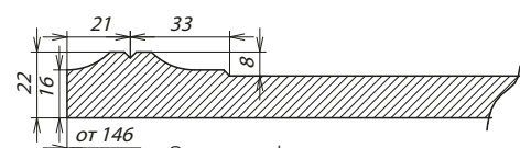
Сечение фасада
