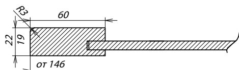
Сечение фасада
