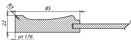
Сечение фасада
