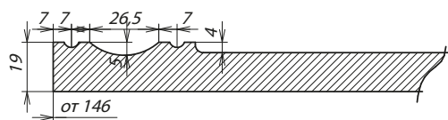
Сечение фасада
