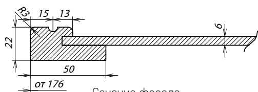
Сечение фасада
