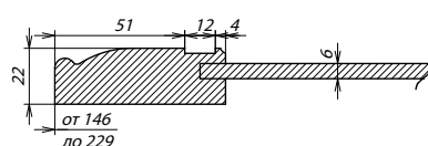
Сечение ПСЯ
