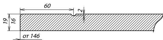
Сечение фасада
