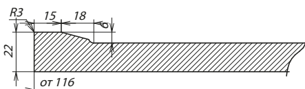
Сечение фасада
