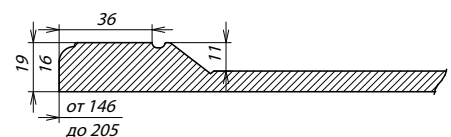
Сечение ПСЯ
