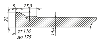
Сечение ПСЯ
